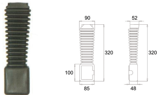
Plastic Gaiter YE 5022 1004
