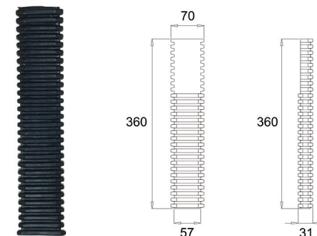
Plastic Gaiter YE 5055 1004
