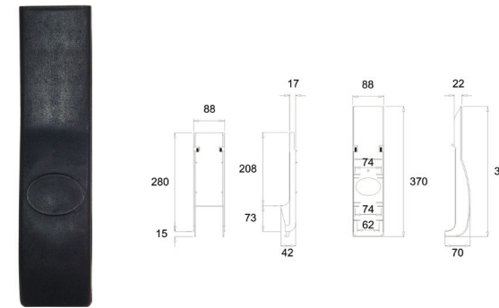
Plastic Gaiter YE 5127 1014
