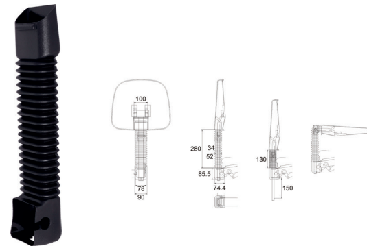
Plastic Gaiter YE 5025 1104
