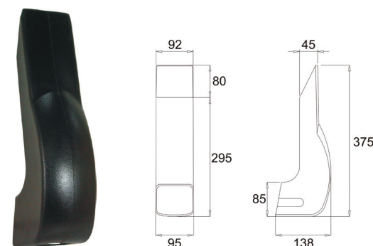
Plastic Gaiter YE 5120 1004
