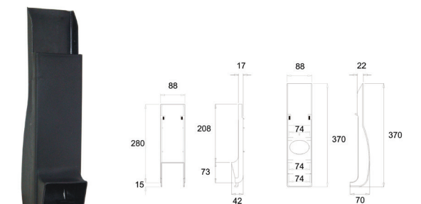
Plastic Gaiter YE 5147 1014
