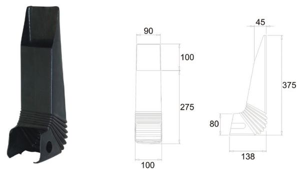
Plastic Gaiter YE 5110 1004
